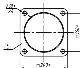
C-C (1:5) A3
